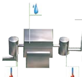
Crystallisation & Separation
